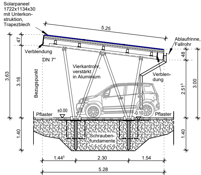
Schnitt A-A
